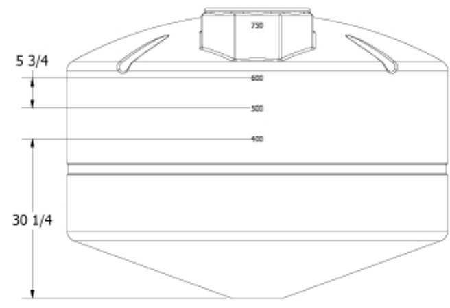
VIEW A-A
